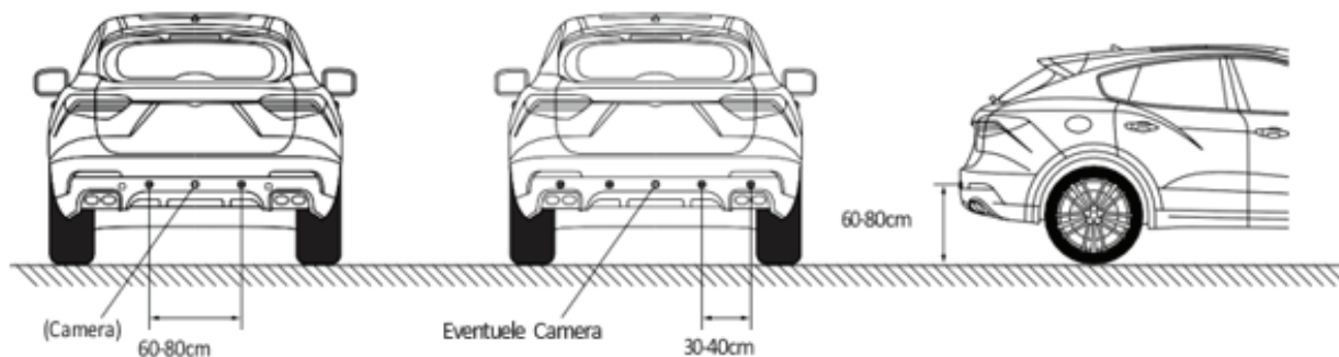
Installatie van de insteeksensoren
