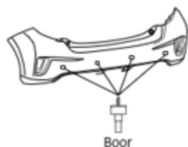
Installatie van de insteeksensoren
